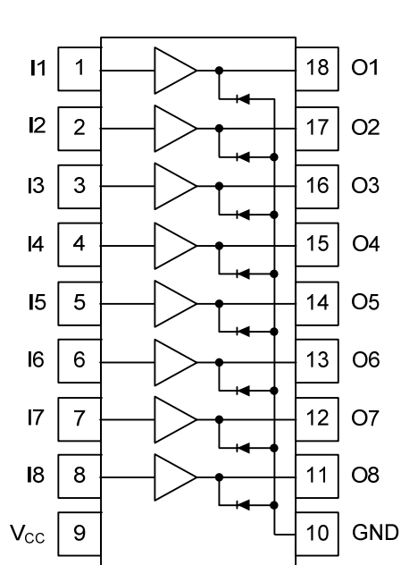
DIP-18 / SOP-18
